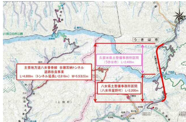
図-1. 合瀬耳納トンネル道路改良事業計画概要図
